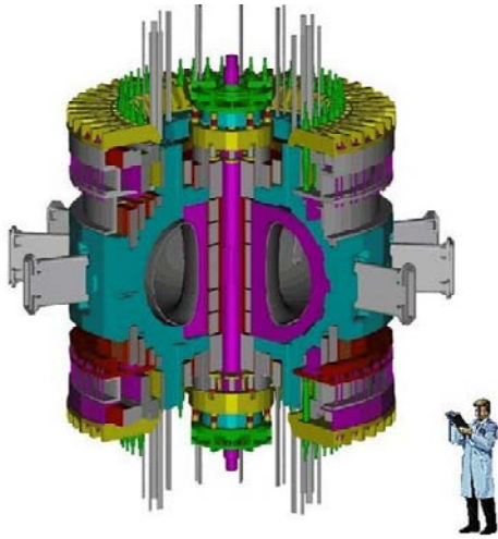
Figura 4. Schizzo di IGNITOR.
