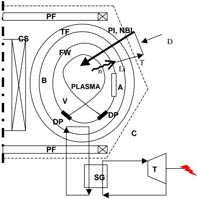
Figura 1. Schizzo di un reattore a fusione di tipo tokamak (sezione verticale passante per l'asse di simmetria della macchina – linea tratto e punto spessa). C = criostato (linea tratteggiata), CS = solenoide centrale, TF = magneti del campo toroidale, PF = magneti del campo poloidale, PI = pellet injector, NBI = neutral beam injector, B = blanket, FW = prima parete, DP = piastra del divertore, A = antenna per il riscaldamento ausiliario (a radiofrequenza) del plasma, V = camera a vuoto (include anche il blanket), SG = generatore di vapore, T = turbina.
